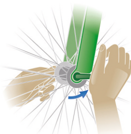
Эксцентрикoвый зажим колесных втулок
